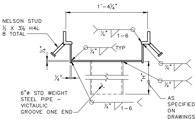
SECTION D-D
