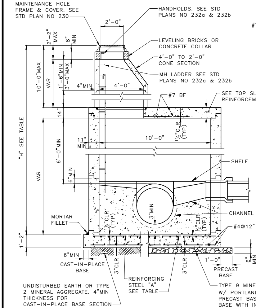
SECTION A-A
