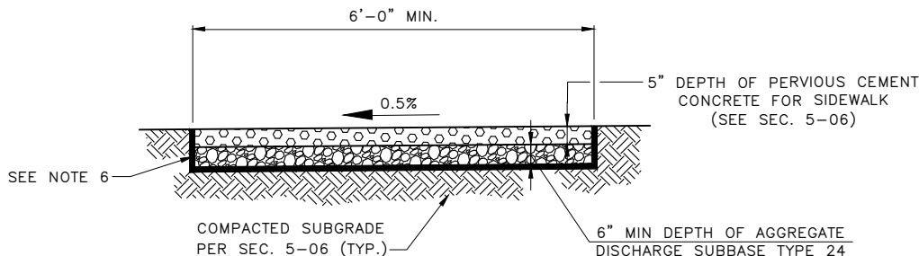
PERVIOUS CONC SECTION A
