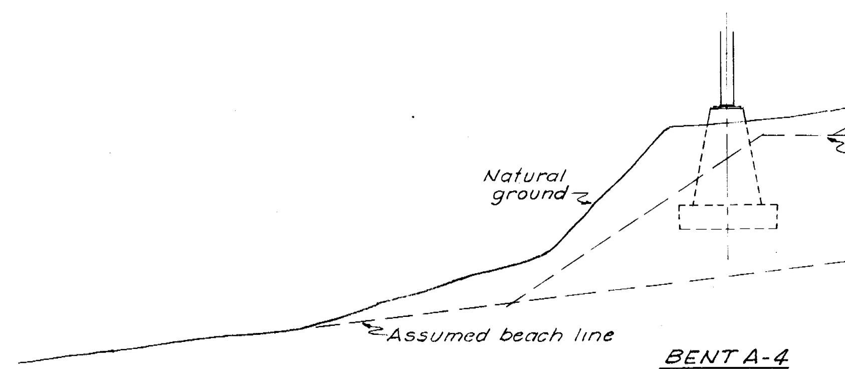
BENT A-4
